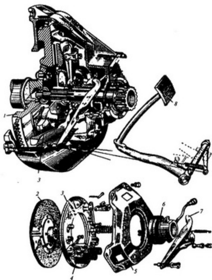
Рис. 2. Clutch
